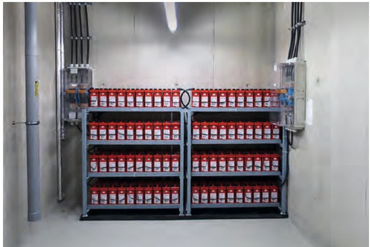
KAT – Garching, USV-Anlage
