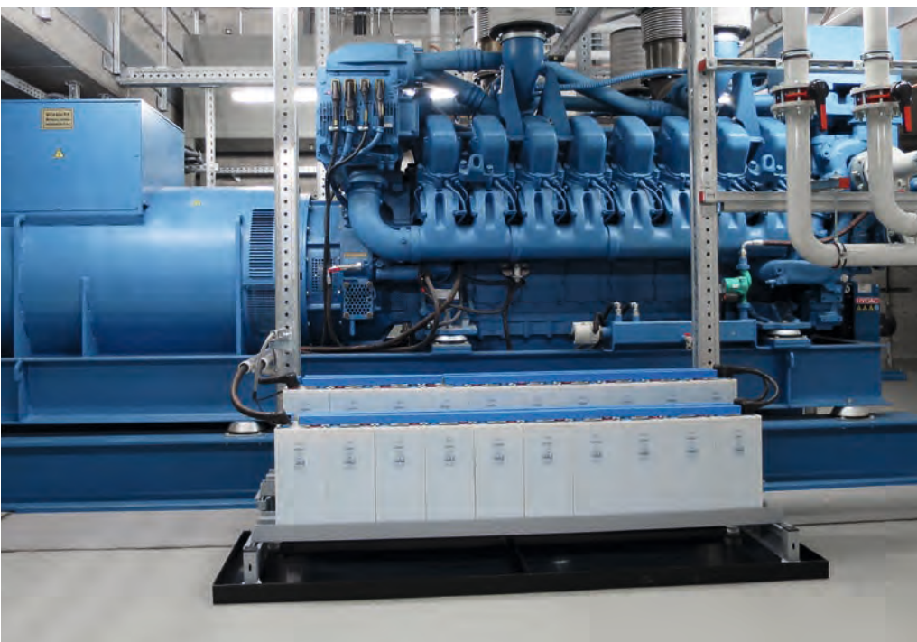
KAT – Garching, Notstromdiesel
